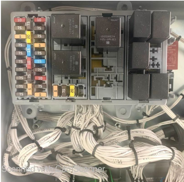
Abbildung 42. Sicherungshalter Sicherungshalters
