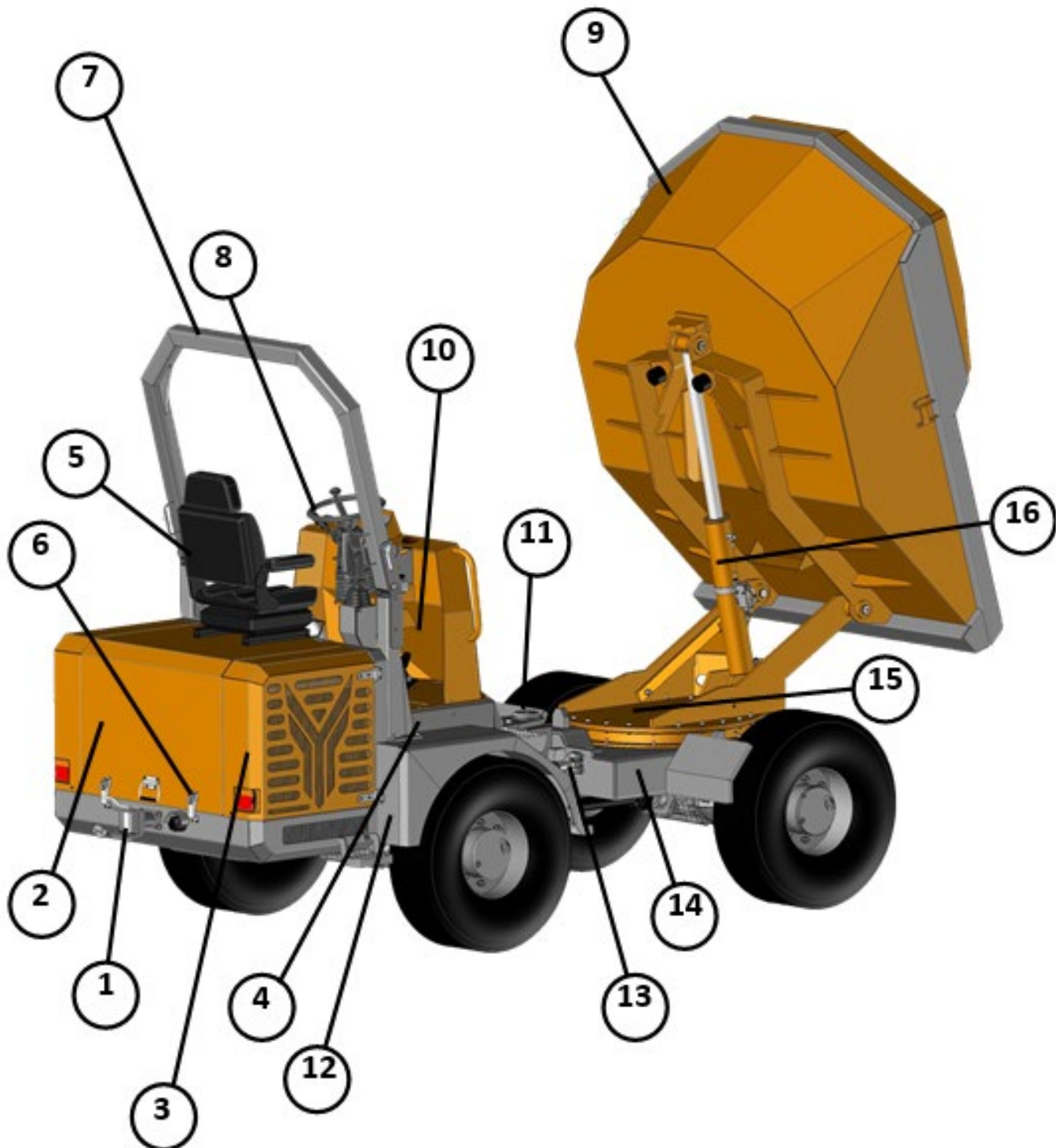
Abbildung 7. Überblick Dumper 4R 1840 RH
