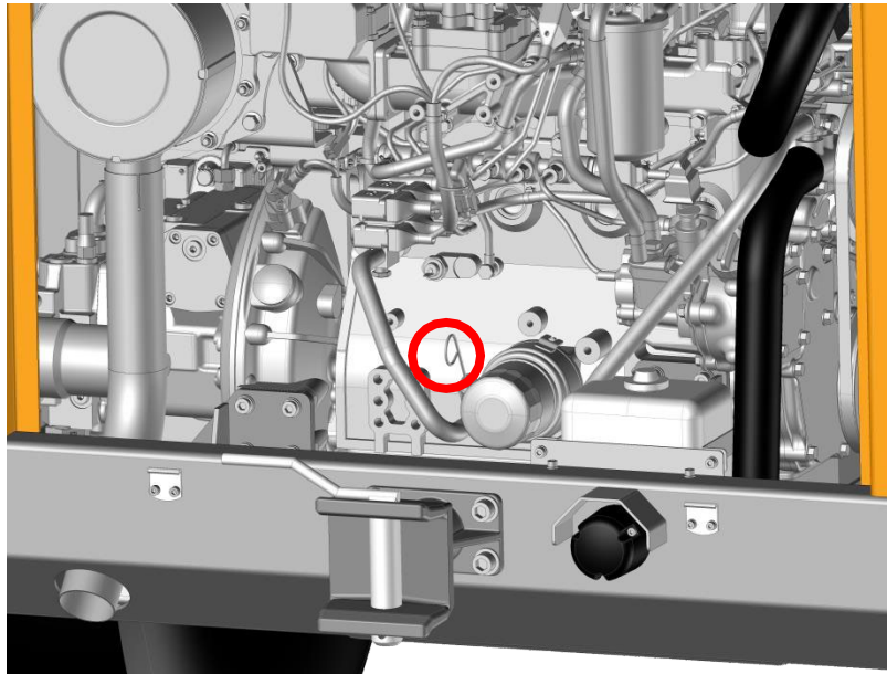
Abbildung 37. Ölmesstab
