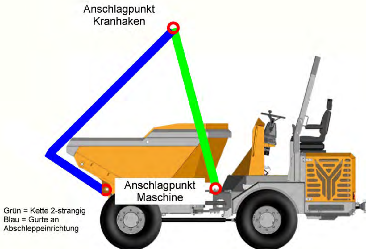
Abbildung 25-L. Kettenanschlagnpunkte an Zugöse auf dem Knickgelenk
