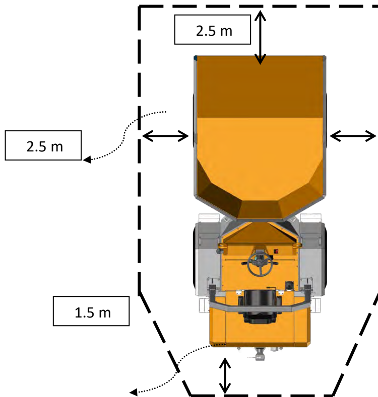
Abbildung 24. Gefahrenbereich
