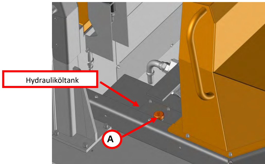
Abbildung 40. Hydrauliköltank
