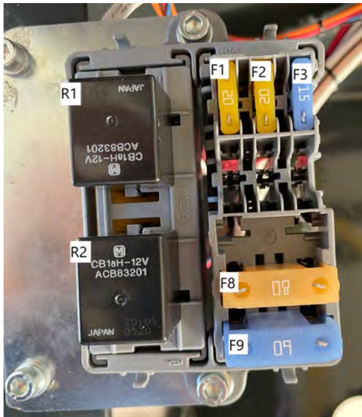
Ansicht Sicherungskasten und Platzierung
