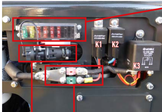
Hauptsicherung
